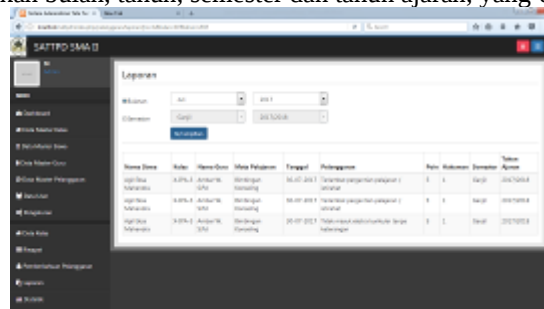
Gambar 20. Halaman Laporan
